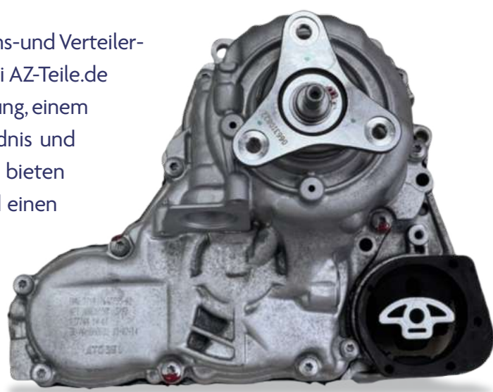
Verteilergetriebe
